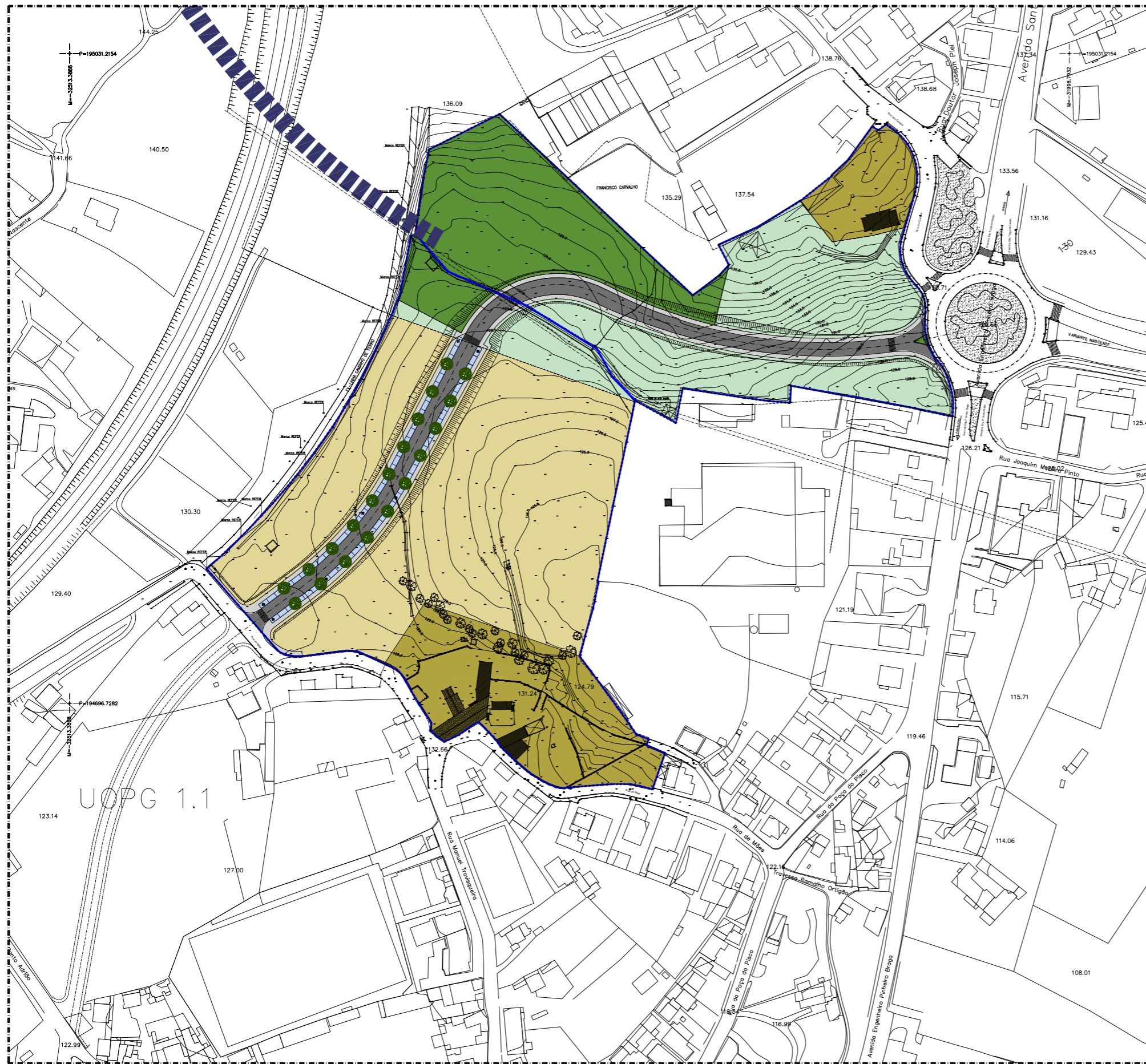
PLANTA DE IMPLANTAÇÃO
