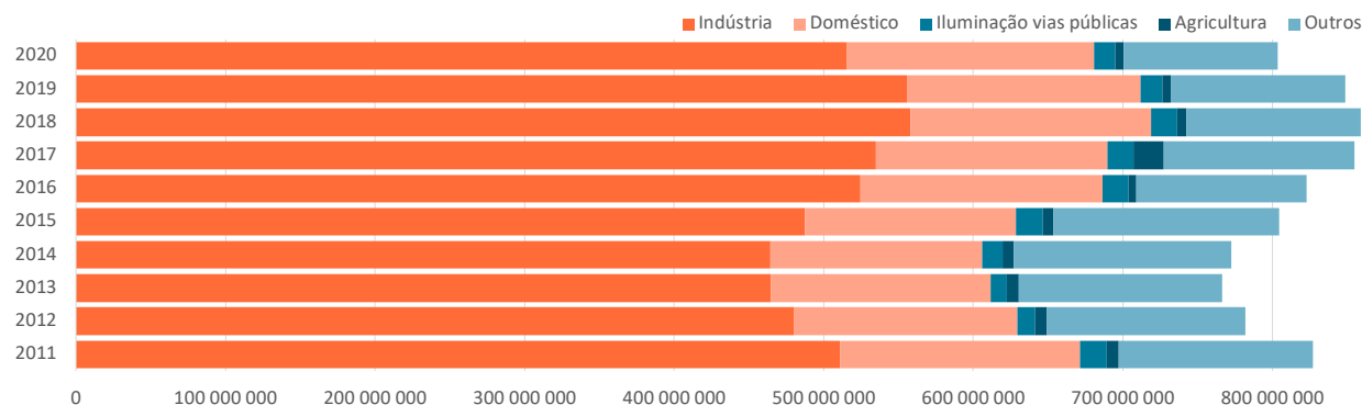
Figura 30- Consumo de energia elétrica em Famalicão (kWh), INE
